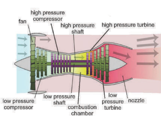
turbo fan
